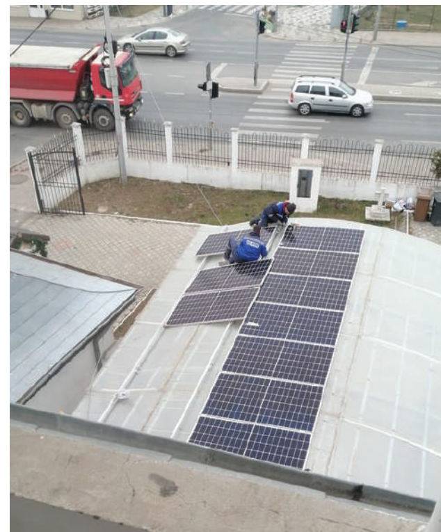
Panouri fotovoltaice la Parohia Chitila III, Șos. Banatului, nr. 14B
